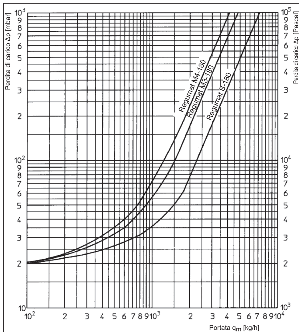
Diagramma delle portate „Regumat-180“
