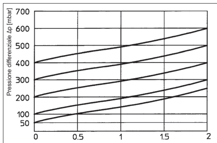
Diagramma delle portate bypass (differenziale)
