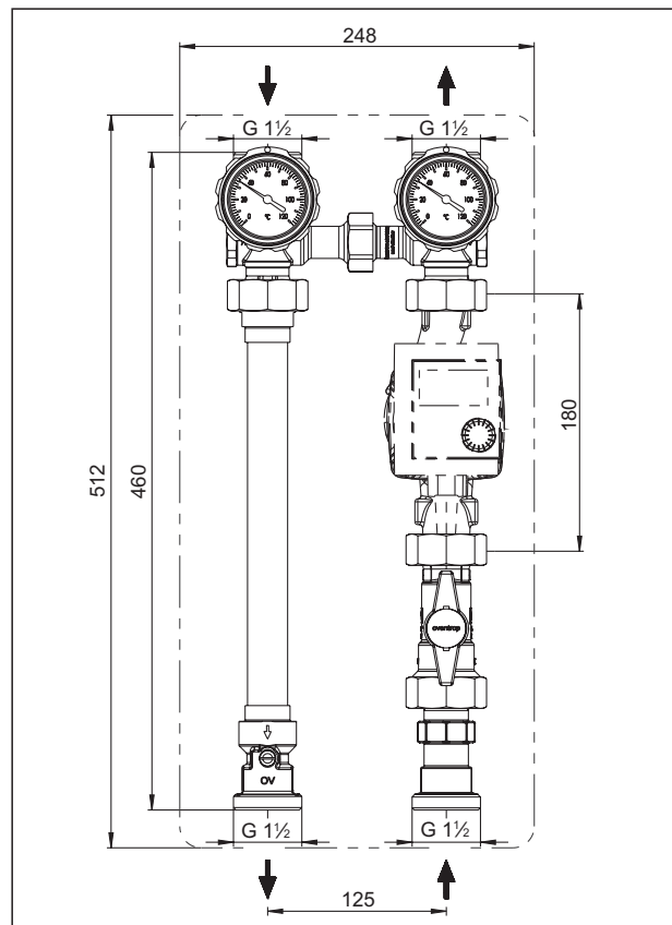
Dimensioni „Regumat S-180“ DN 25 con valvola a sfera per pompa installata prima della pompa
