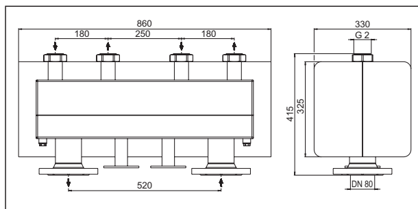
Dimensioni „HydroFixx“ DN 40/50, 2 circuiti
