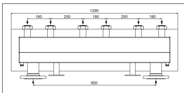
Dimensioni „HydroFixx“ DN40/50, 3 circuiti
