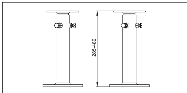
Dimensioni set piedini
