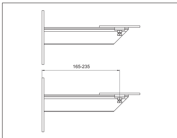
Dimensioni set mensole per fissaggio a muro
