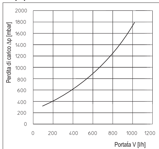
Perdita di carico circuito acqua sanitaria – Campo prestazionale 2
