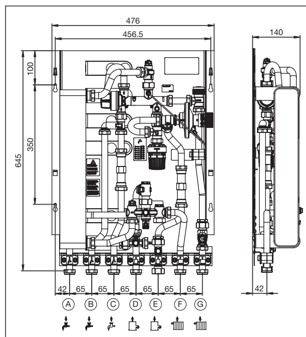
Dimensioni
