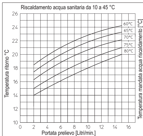
Temperatura ritorno – Campo prestazionale 2 – 15 l/min
