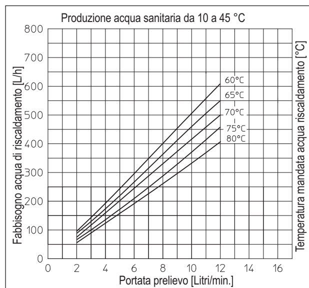
Fabbisogno acqua calda – Campo prestazionale 1 – 12 l/min
