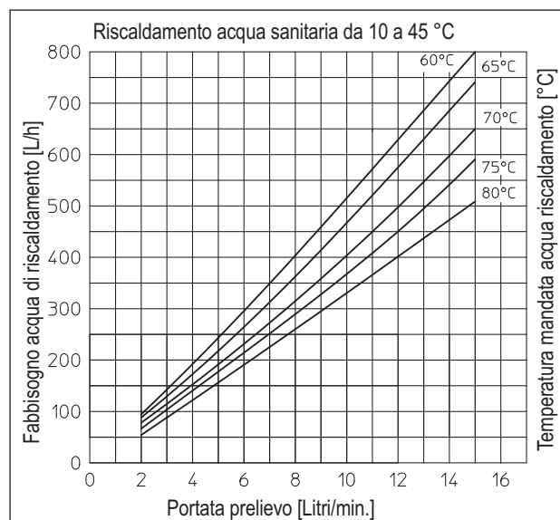
Fabbisogno acqua calda – Campo prestazionale 2 – 15 l/min
