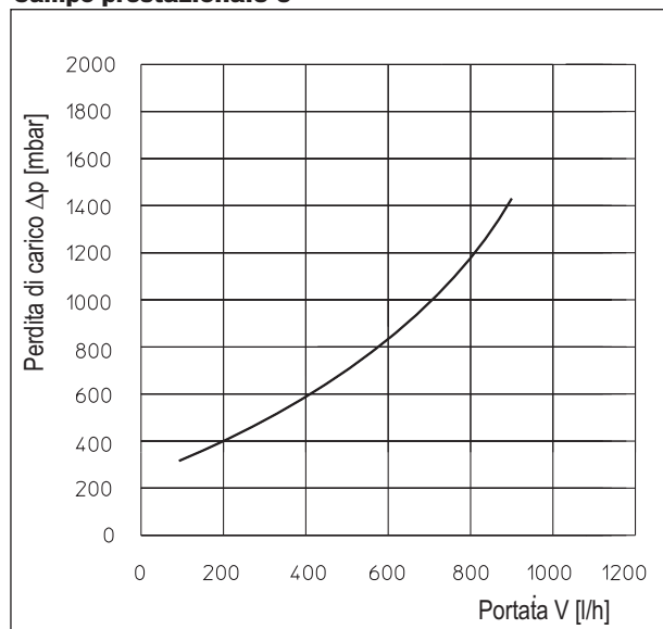
Perdita di carico circuito riscaldamento
