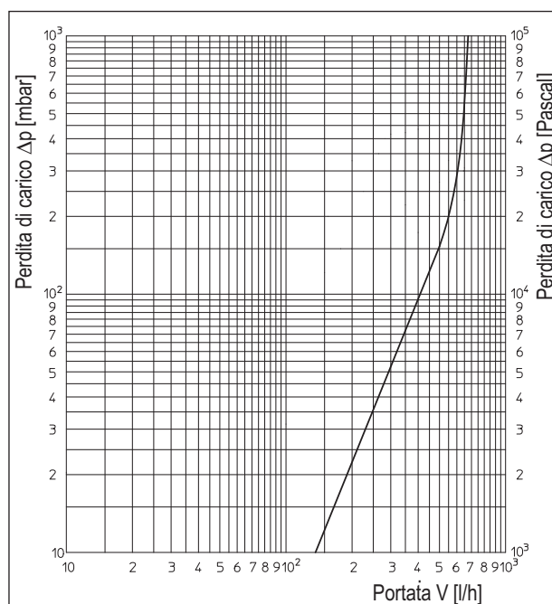
Perdita di carico circuito riscaldamento
