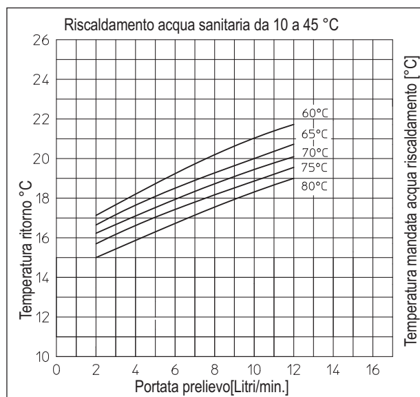
Temperatura ritorno – Campo prestazionale 1 – 12 l/min
