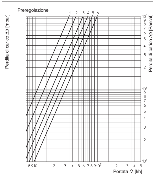
„Aquastrum VT“ DN 15 portata residua
