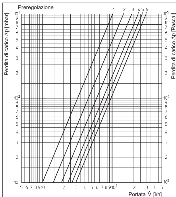
„Aquastrum VT“ DN 20 Portata residua
