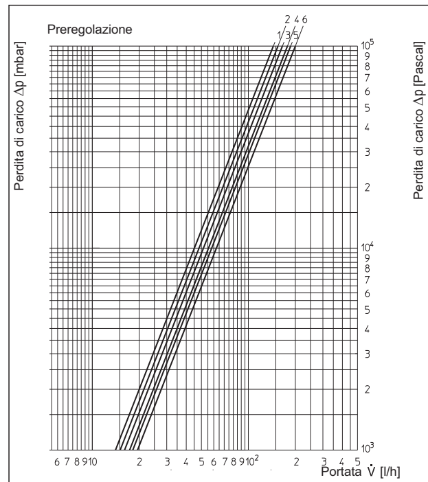
„Aquastrum VT“ DN 15 portata di disinfezione
