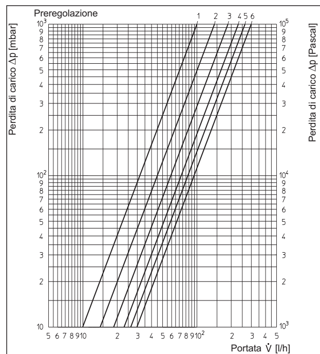
„Aquastrum VT“ DN 20 Portata di disinfezione
