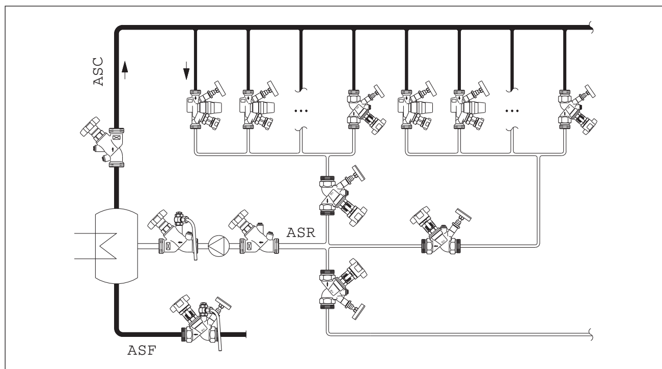
Schema impianto
