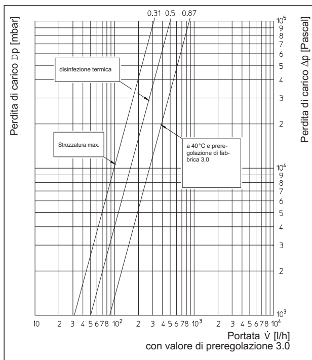
„Aquamstrom T plus“ DN 20
