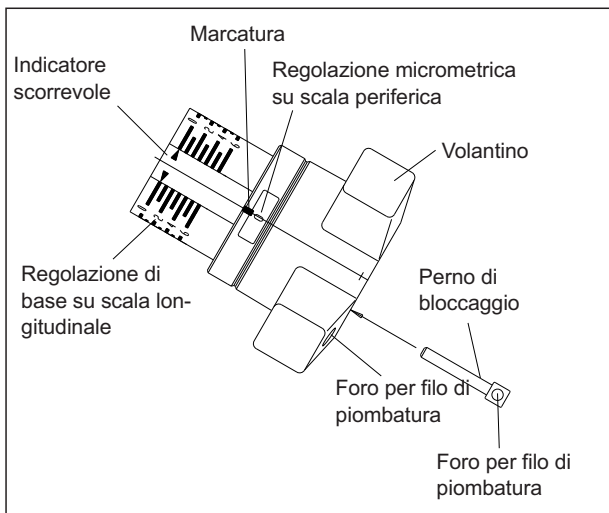
Azionamento manuale
