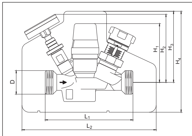
„Aquastrom T plus“
